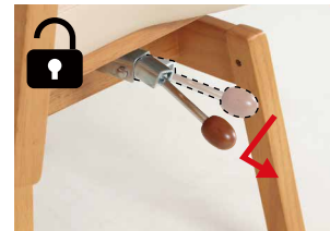
レバーを下げて引っぱると90°ロックが解除になり、360°回転します。
